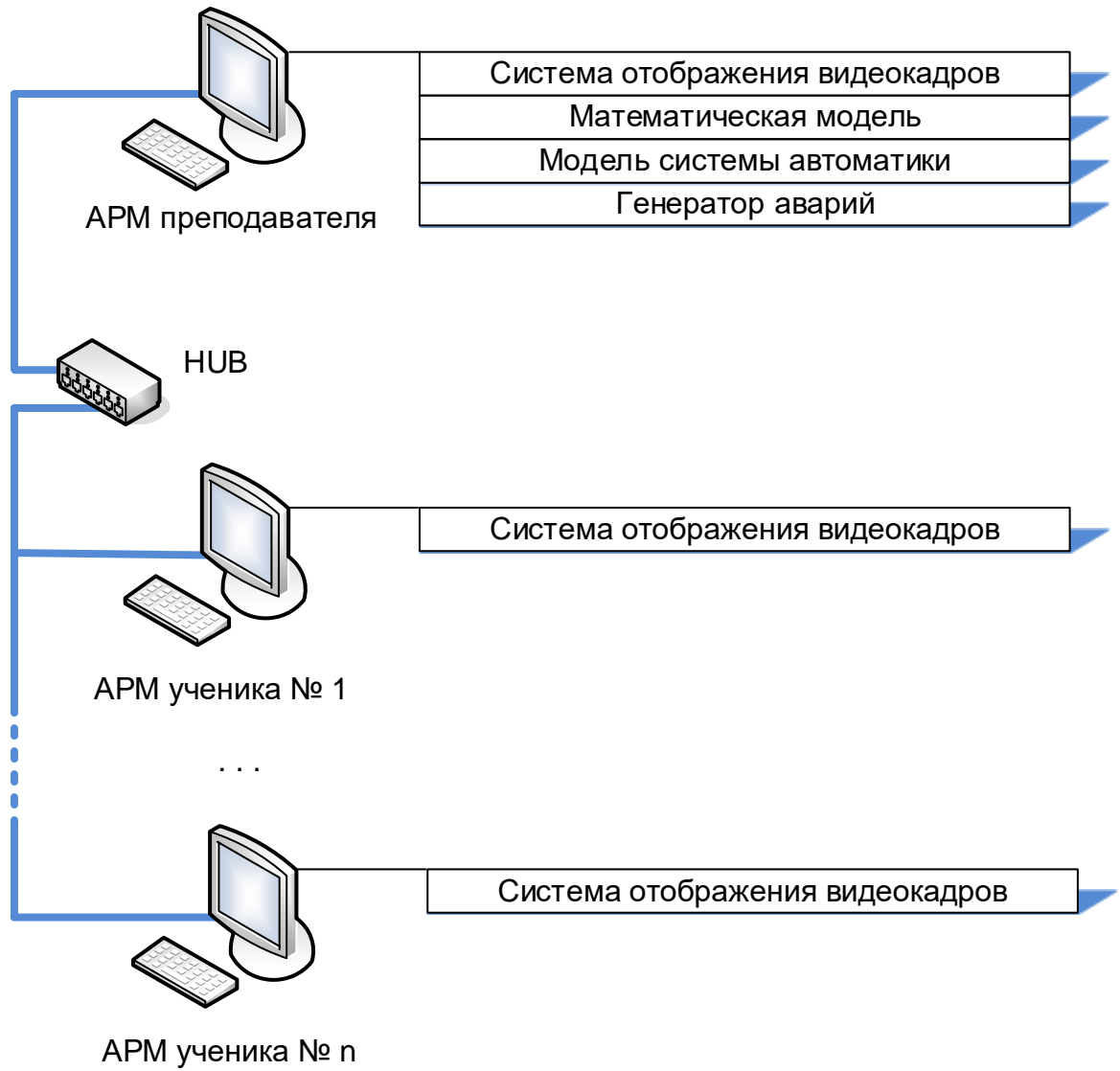
Рисунок 1.1 Структурная схема ПО Тренажера
